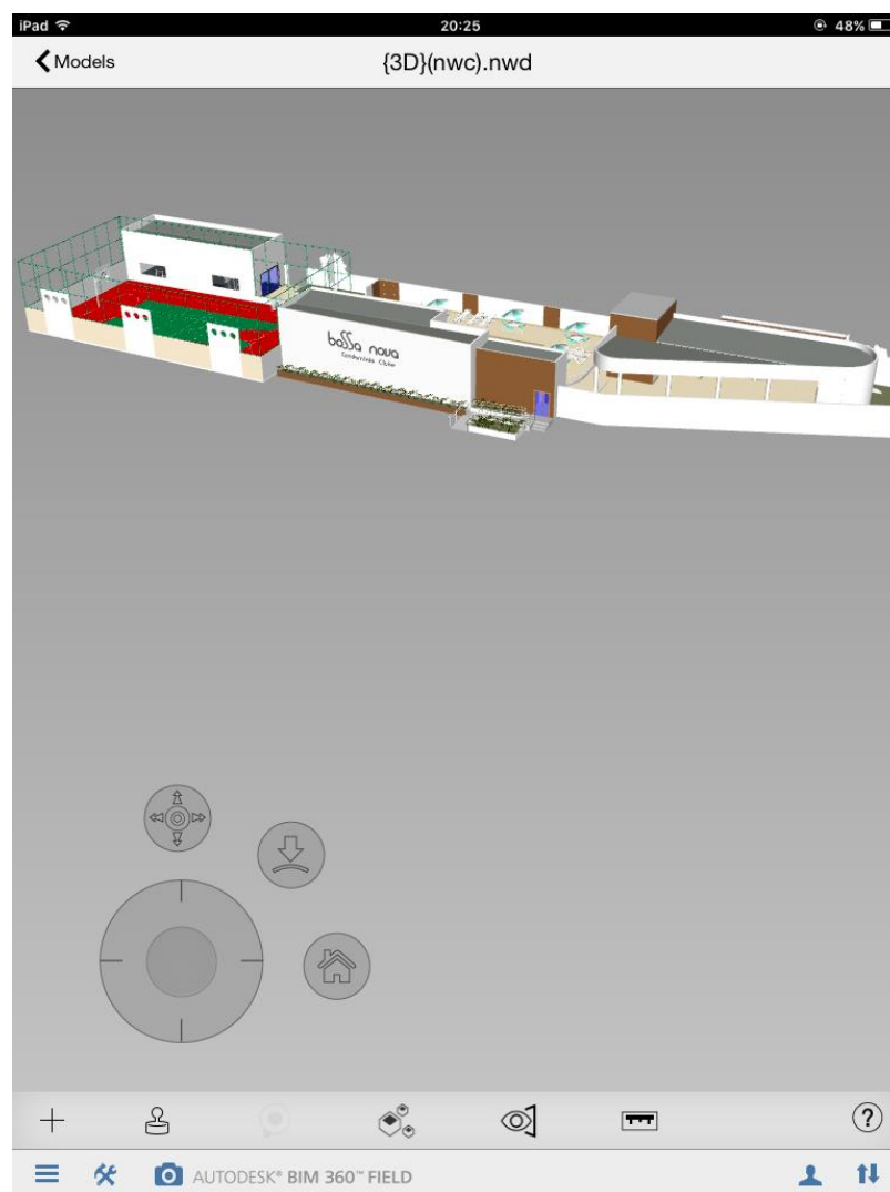
Figura 10 – Modelo arquitetônico no iPad.
