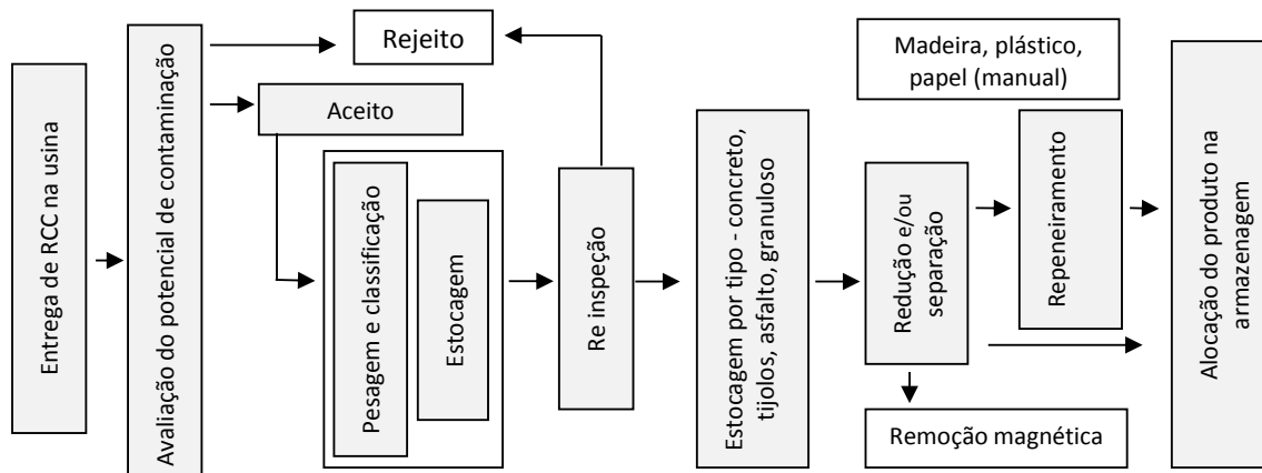
Figura 1 - Método de controle em usinas na Europa
