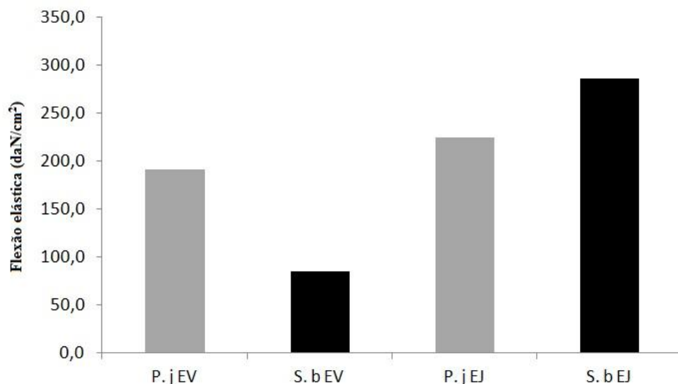
Gráfico 2.4.11. Valores médios de flexão elástica para as estacas velhas e jovens de P. juliflora e S. brasiliensis .
